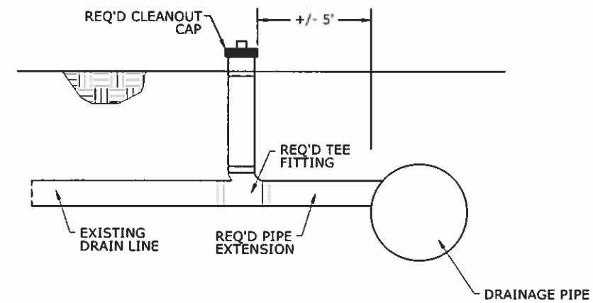
SEWER EFFLUENT PIPE TIE-IN
